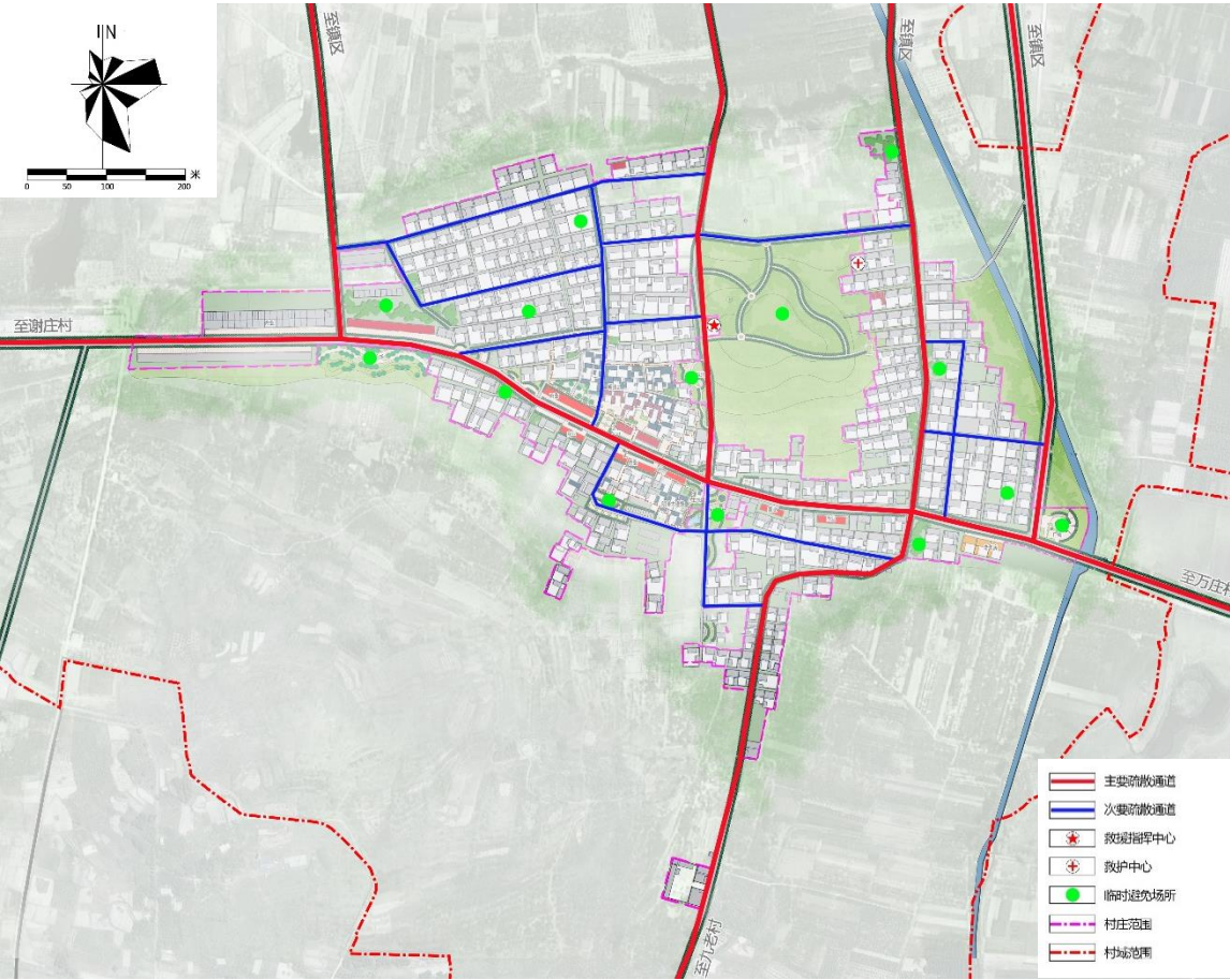
图7—7 综合防灾规划图
