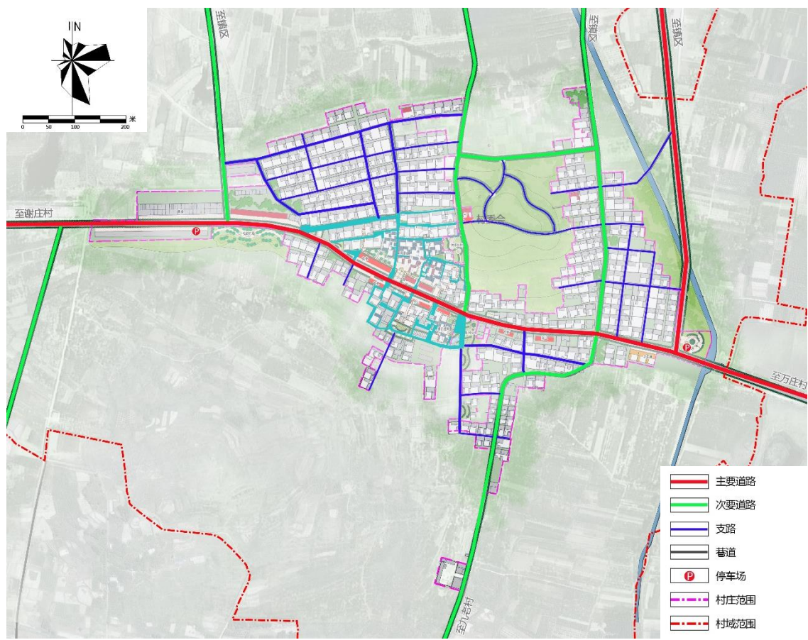
图7—3 水山村道路交通规划图
