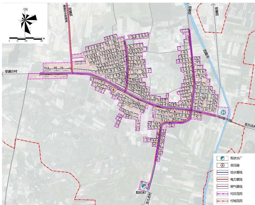
图2—4 基础设施建设现状图
