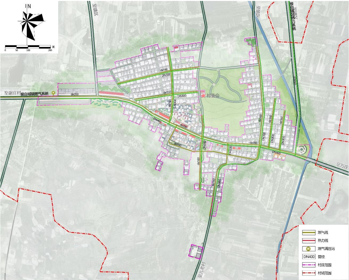
图7—6 热力燃气规划图
