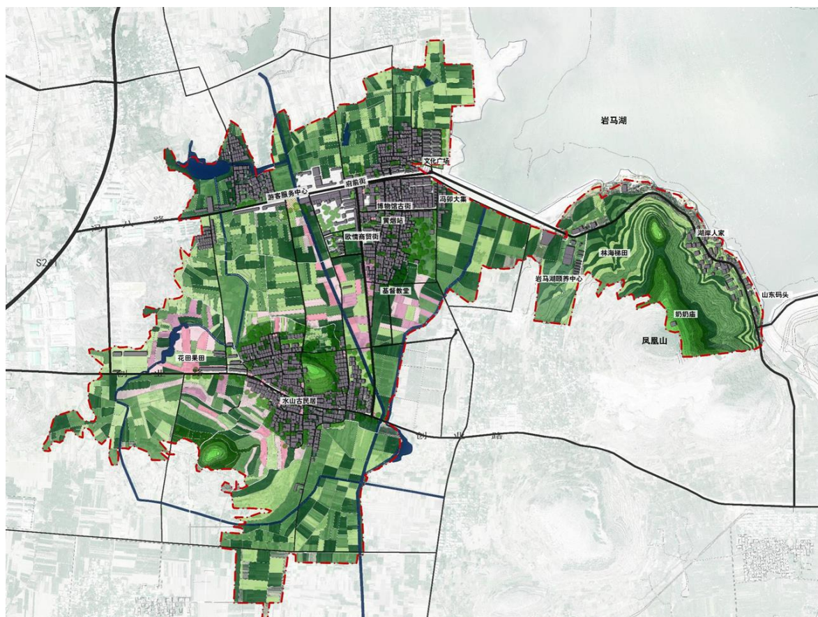
图1-2 规划平面图
