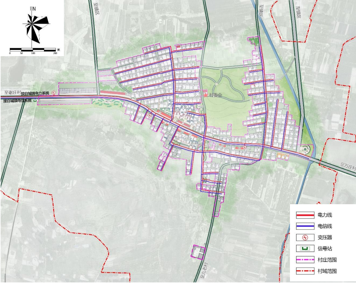
图7—5 电力电信规划图
