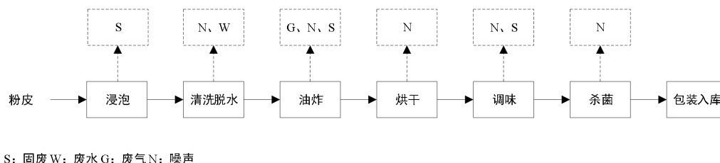
图 2-4 风味粉皮生产工艺流程及产污环节图
