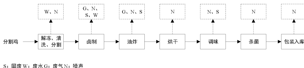
图 2-3 鸡肉熟食生产工艺流程及产污环节图
