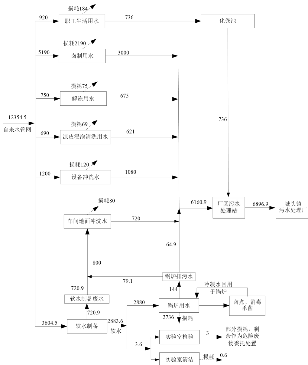
图 2-1 项目全厂水平衡图 (t/a)
